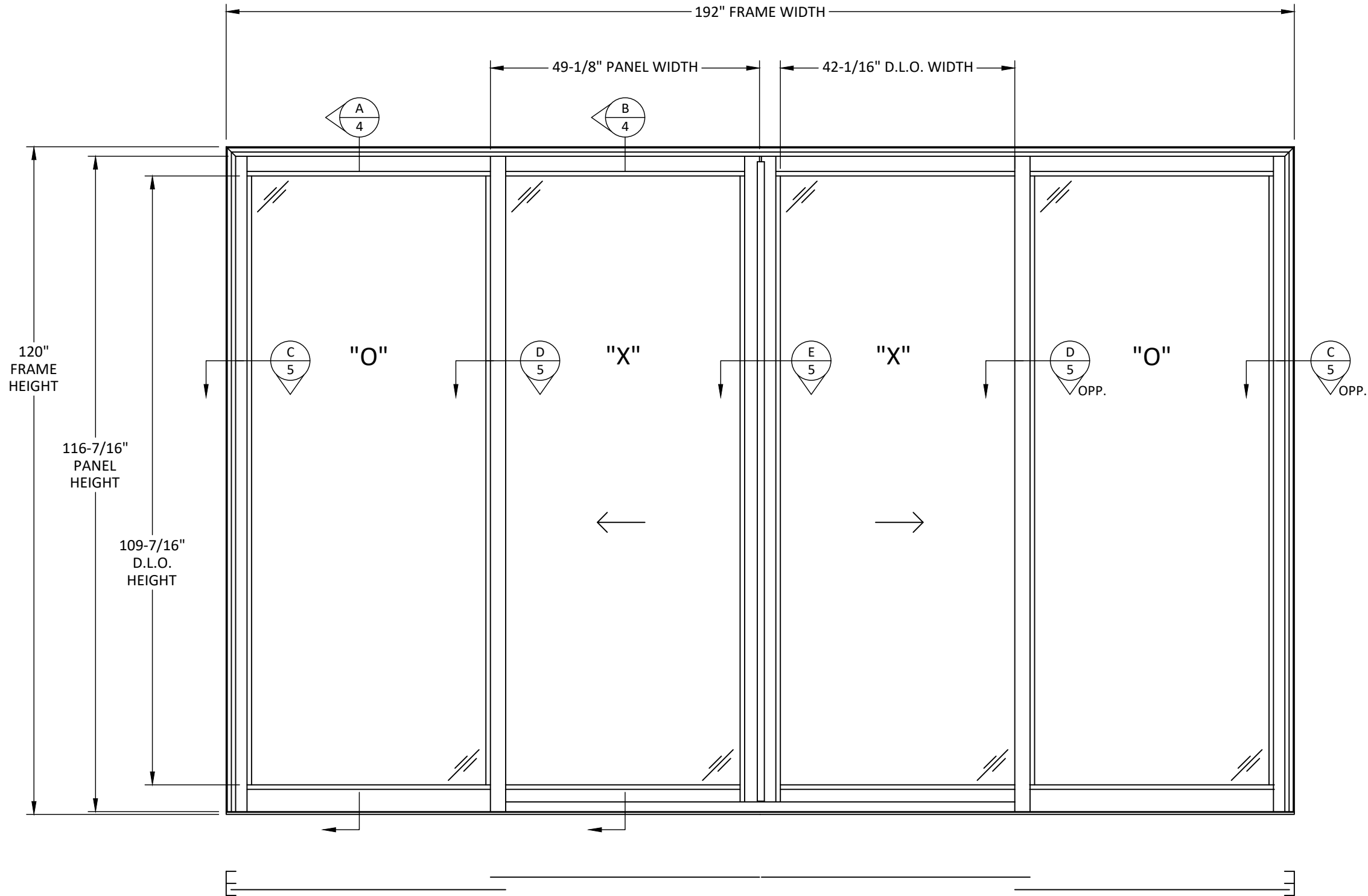
ELEVATION OX XO
